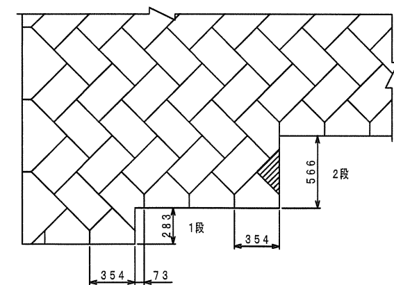
段違い配置参考図
